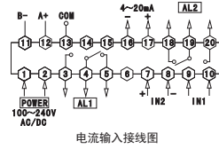
电流输入接线图
