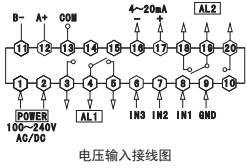
电压输入接线图
